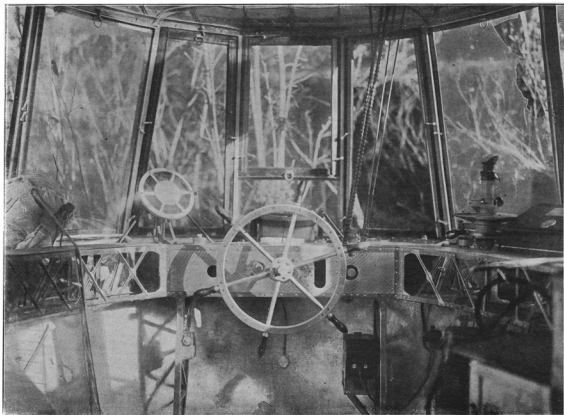
Poste de commandement, dans la nacelle avant du L. 49, descendu à Bourbonne-les-Bains.
